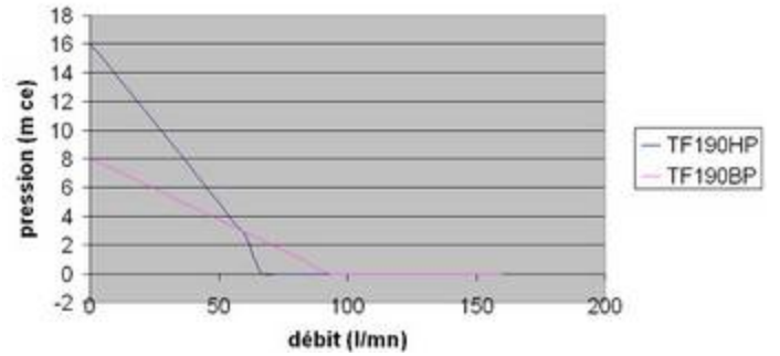
POMPE VIDE FUT TECHNI-FLOW TF190HP/TF190BP
